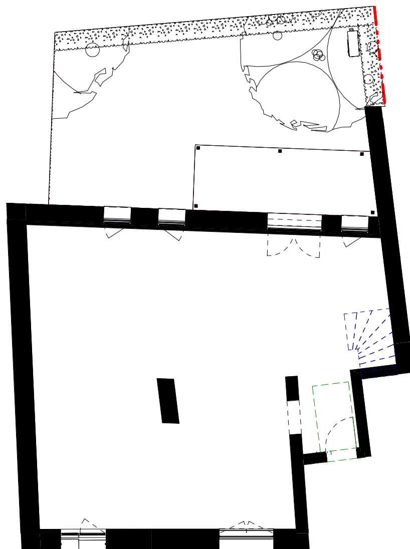
REZ-DE-CHAUSSÉE
