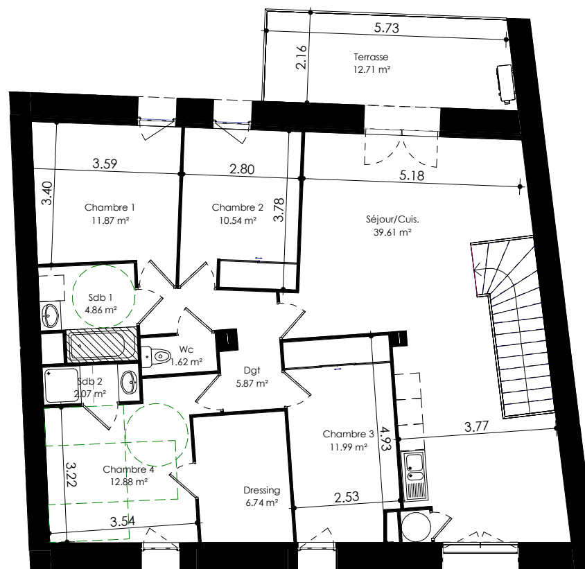
ÉTAGE
