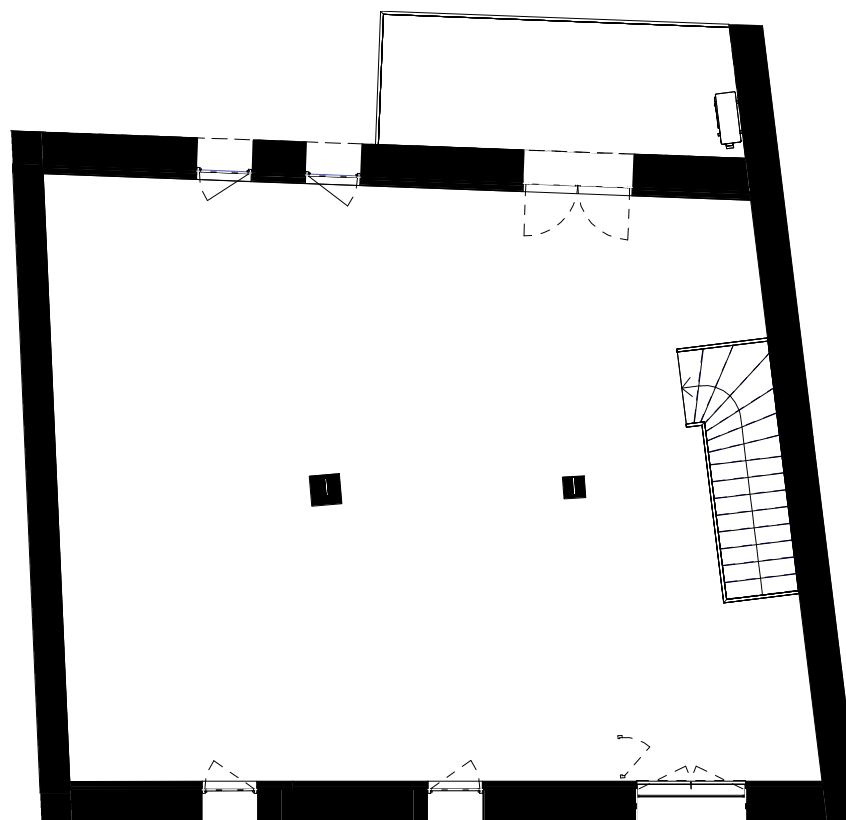
ÉTAGE
